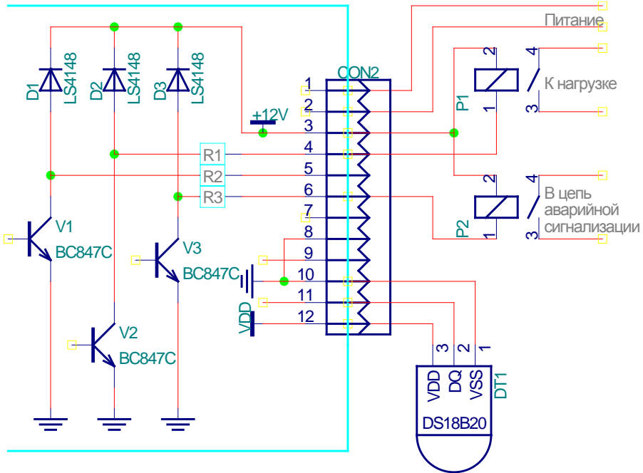
Рис. 1. (Подключение контроллера).
