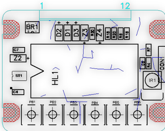
Вид сверху
